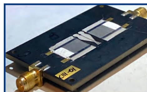
Лабораторный макет
